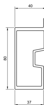
groefprofiel
