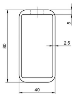
midden profiel
