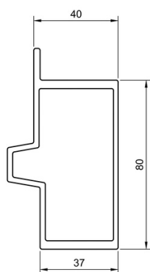
tandprofiel
